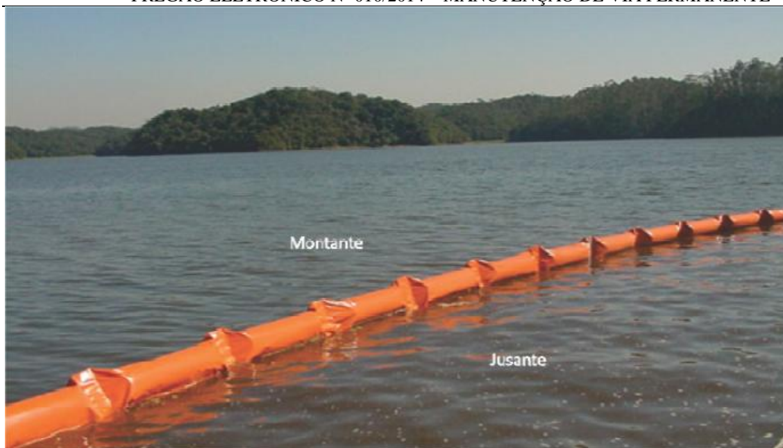
Figura 1 - Modelo de barreira retentora de óleo
